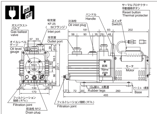
サーマルプロテクター内蔵 (手動復帰) With built-in thermal protector
